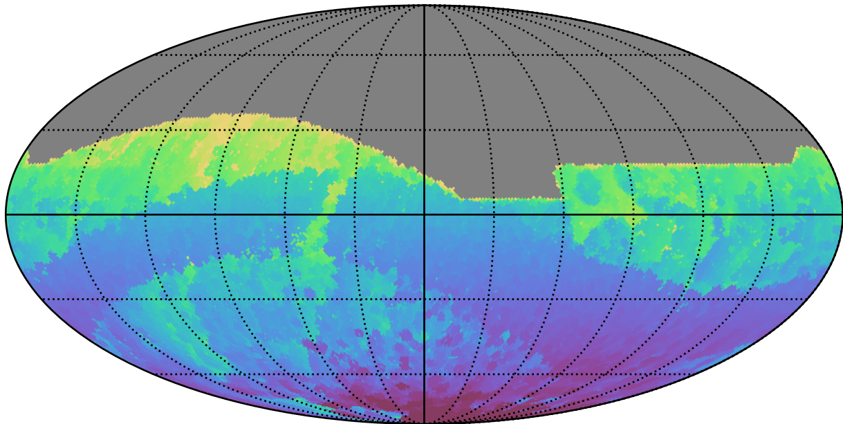
no_magell_roll_v3.4_10yrs All sky r band: Min HA
