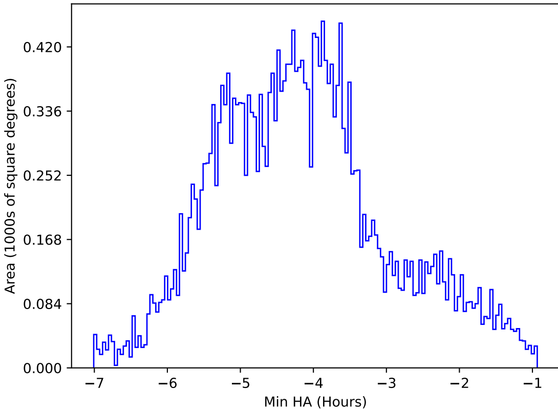
no_magell_roll_v3.4_10yrs All sky r band: Min HA
