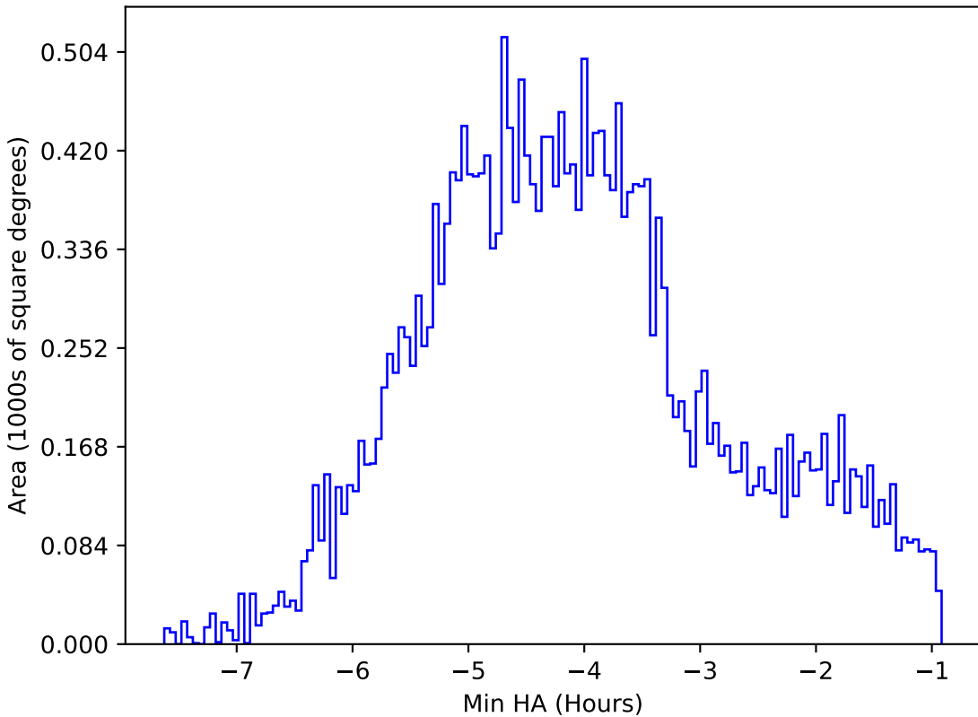
no_magell_roll_v3.4_10yrs All sky i band: Min HA
