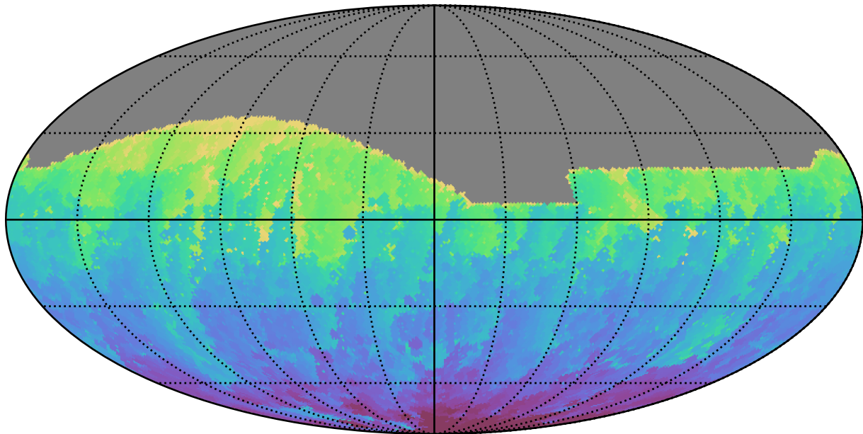
no_magell_roll_v3.4_10yrs All sky g band: Min HA
