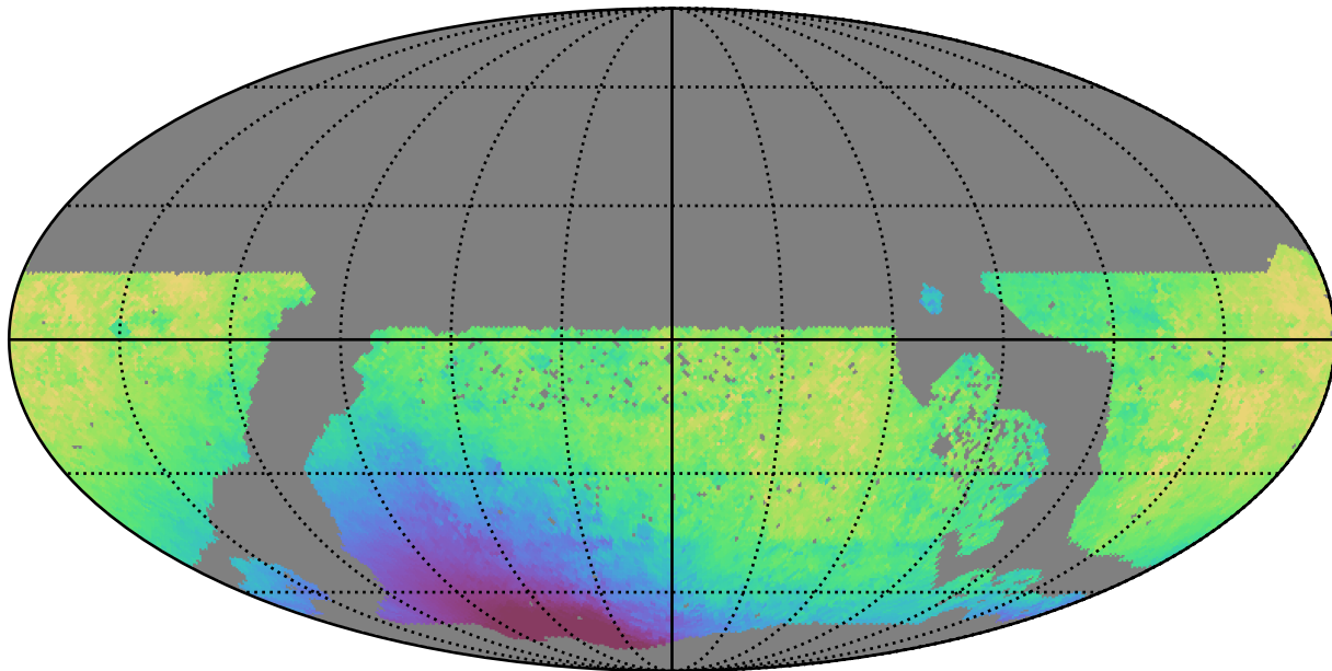
no_magell_roll_v3.4_10yrs WFD y band: Median solarElong
