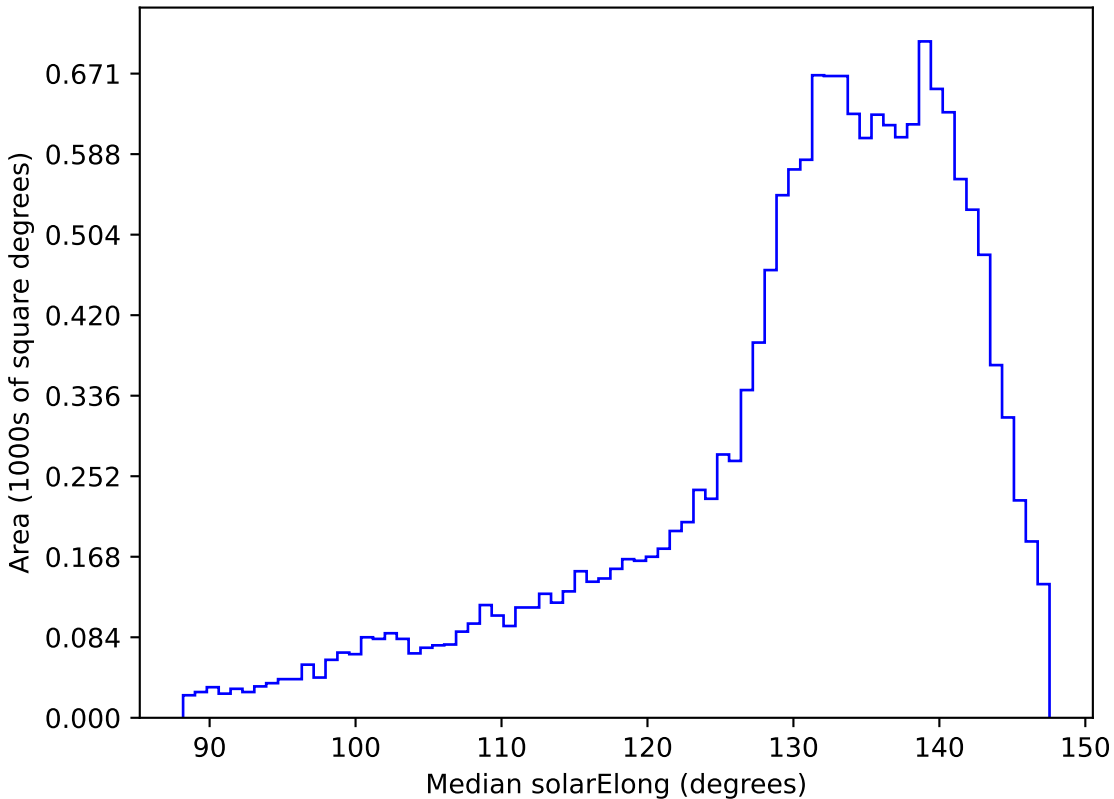
no_magell_roll_v3.4_10yrs WFD y band: Median solarElong
