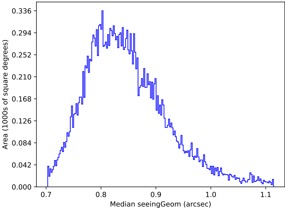
no_magell_roll_v3.4_10yrs Yr 1 y band: Median seeingGeom
