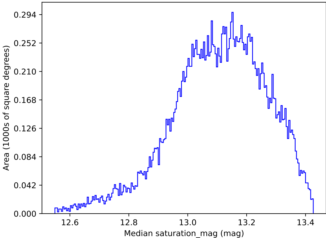
no_magell_roll_v3.4_10yrs All sky y band: Median saturation_mag
