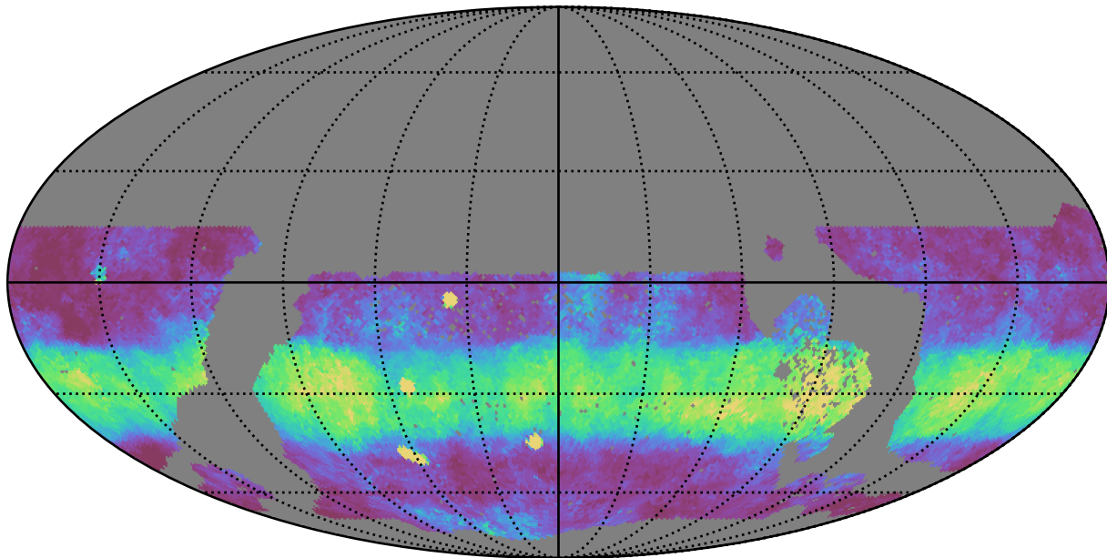
no_magell_roll_v3.4_10yrs WFD y band: Median normairmass
