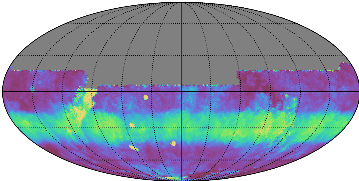
no_magell_roll_v3.4_10yrs All sky y band: Median normairmass
