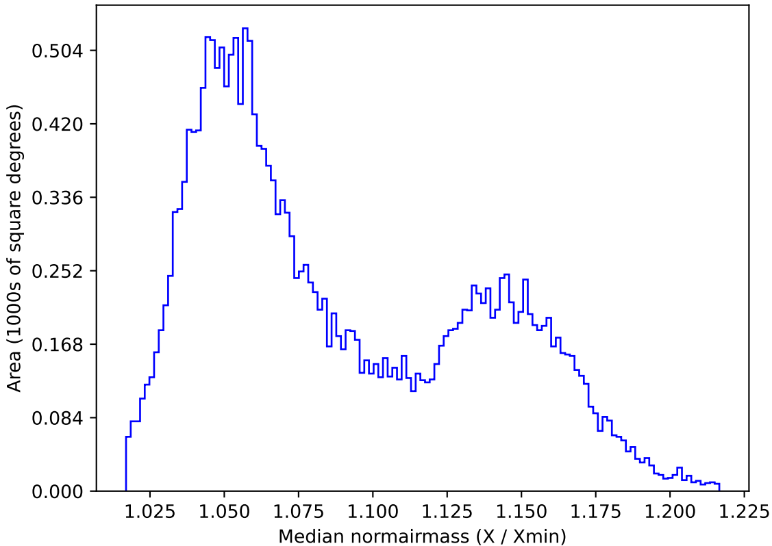
no_magell_roll_v3.4_10yrs All sky y band: Median normairmass
