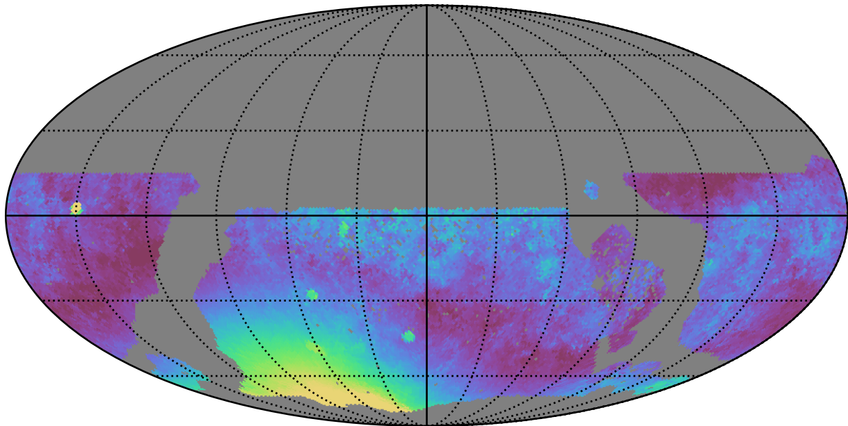
no_magell_roll_v3.4_10yrs WFD y band: Median moonDistance
