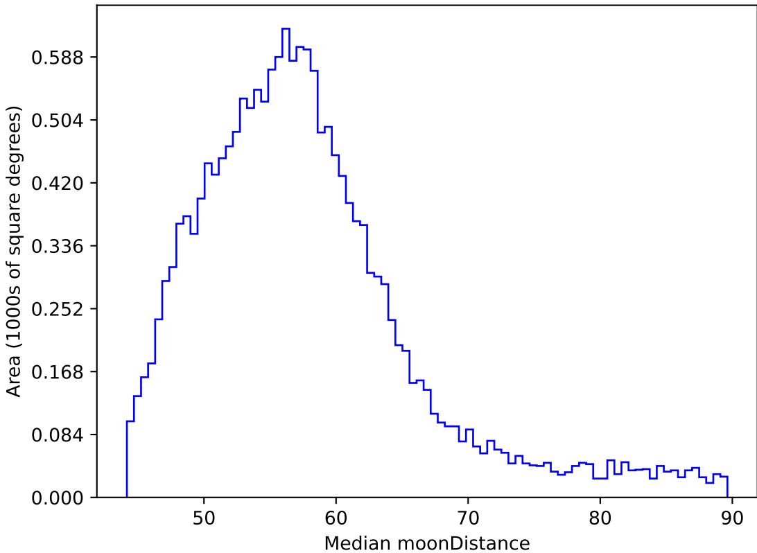
no_magell_roll_v3.4_10yrs WFD y band: Median moonDistance
