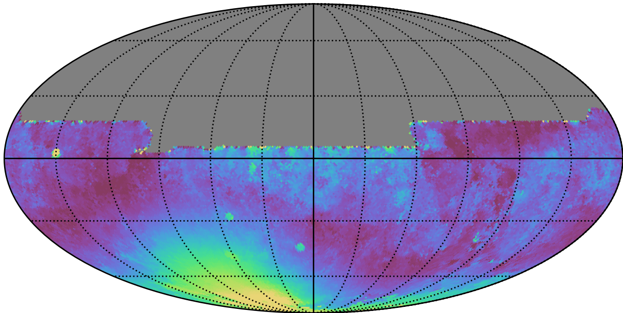
no_magell_roll_v3.4_10yrs All sky y band: Median moonDistance
