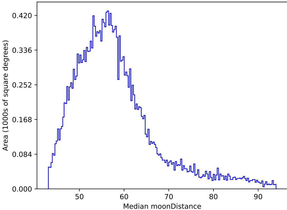
no_magell_roll_v3.4_10yrs All sky y band: Median moonDistance
