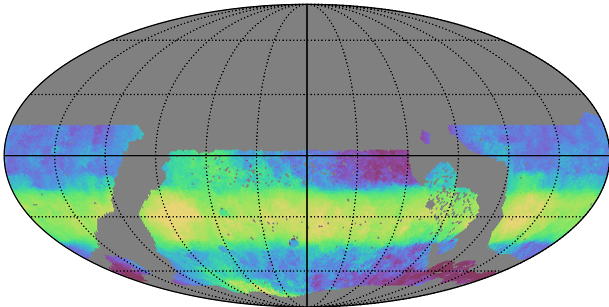
no_magell_roll_v3.4_10yrs WFD z band: Median HA
