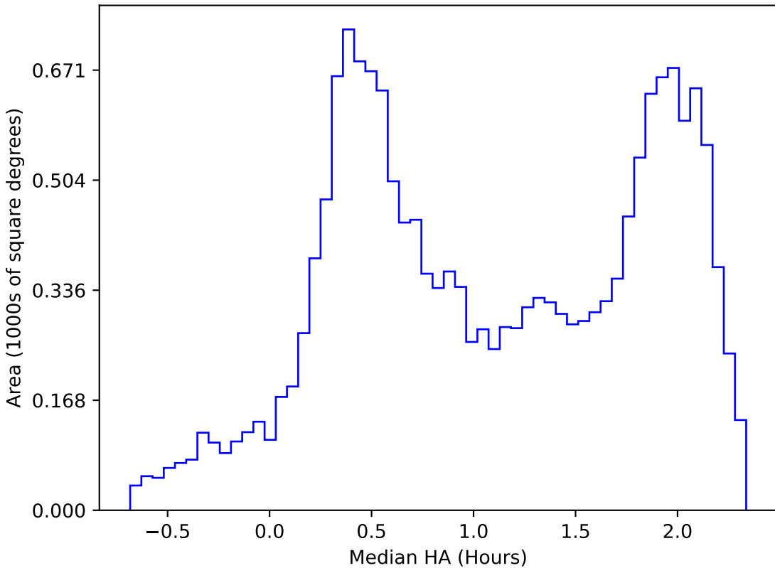
no_magell_roll_v3.4_10yrs WFD z band: Median HA
