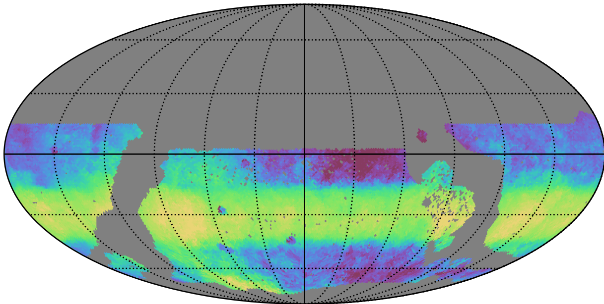
no_magell_roll_v3.4_10yrs WFD y band: Median HA
