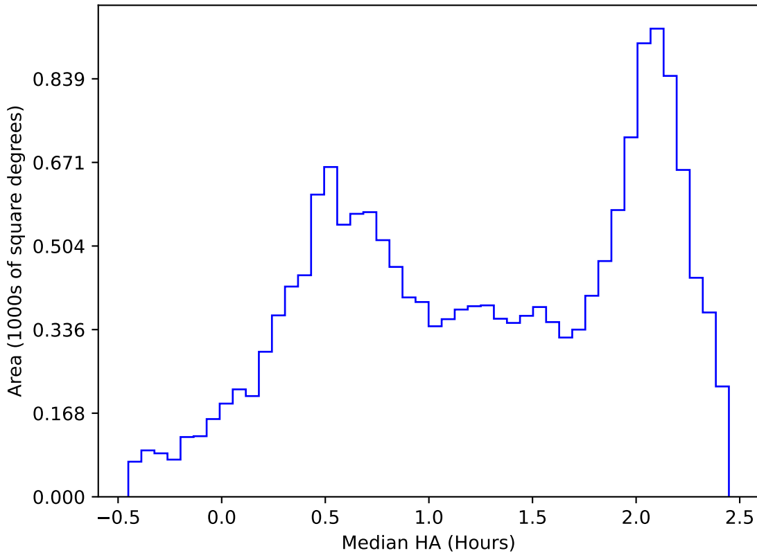
no_magell_roll_v3.4_10yrs WFD y band: Median HA
