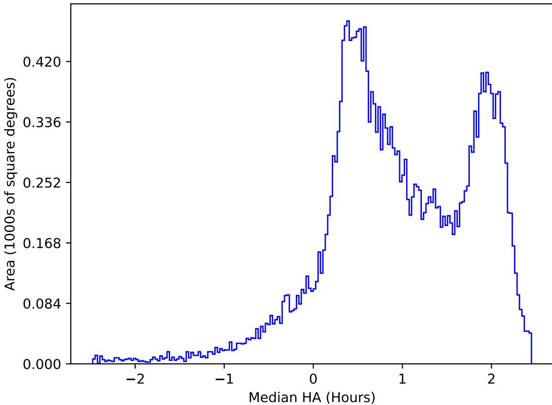
no_magell_roll_v3.4_10yrs All sky z band: Median HA
