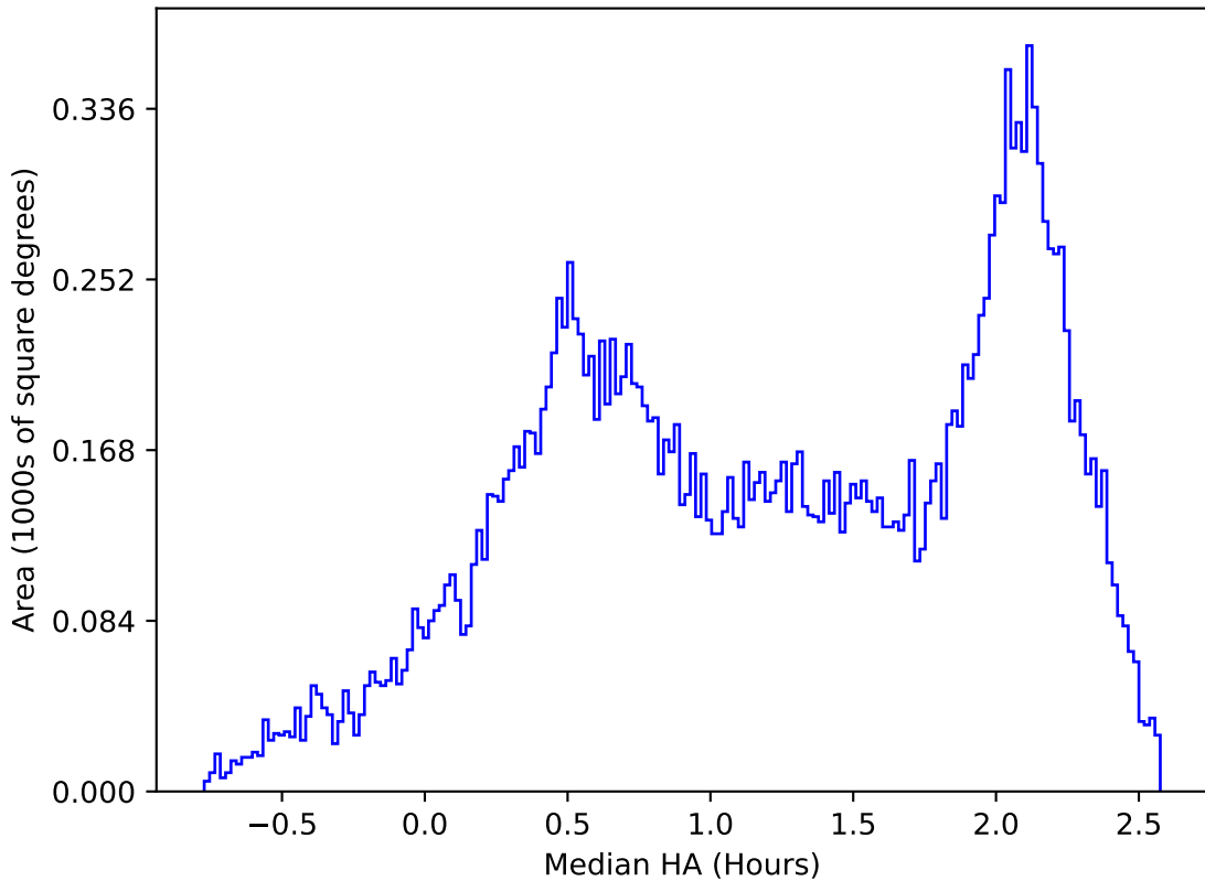
no_magell_roll_v3.4_10yrs All sky y band: Median HA
