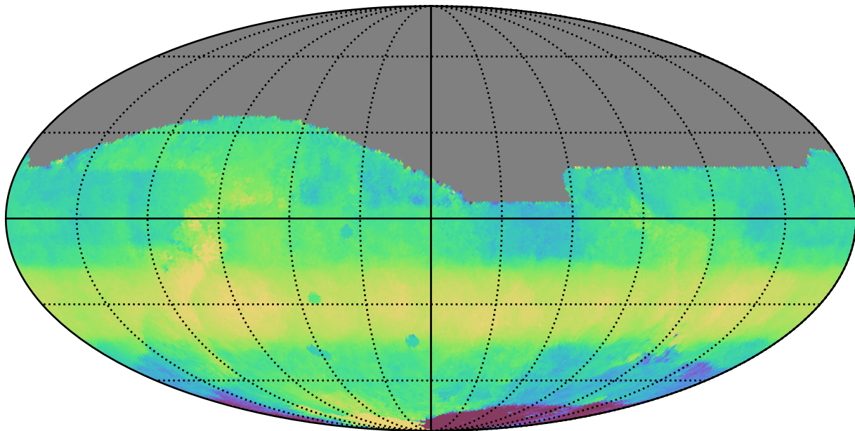
no_magell_roll_v3.4_10yrs All sky i band: Median HA
