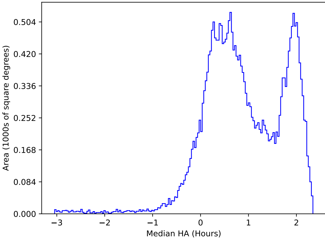
no_magell_roll_v3.4_10yrs All sky i band: Median HA
