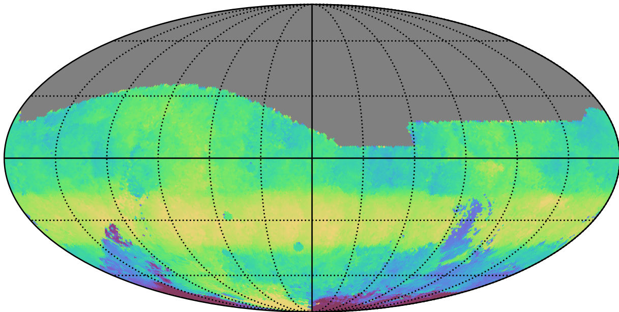
no_magell_roll_v3.4_10yrs All sky g band: Median HA
