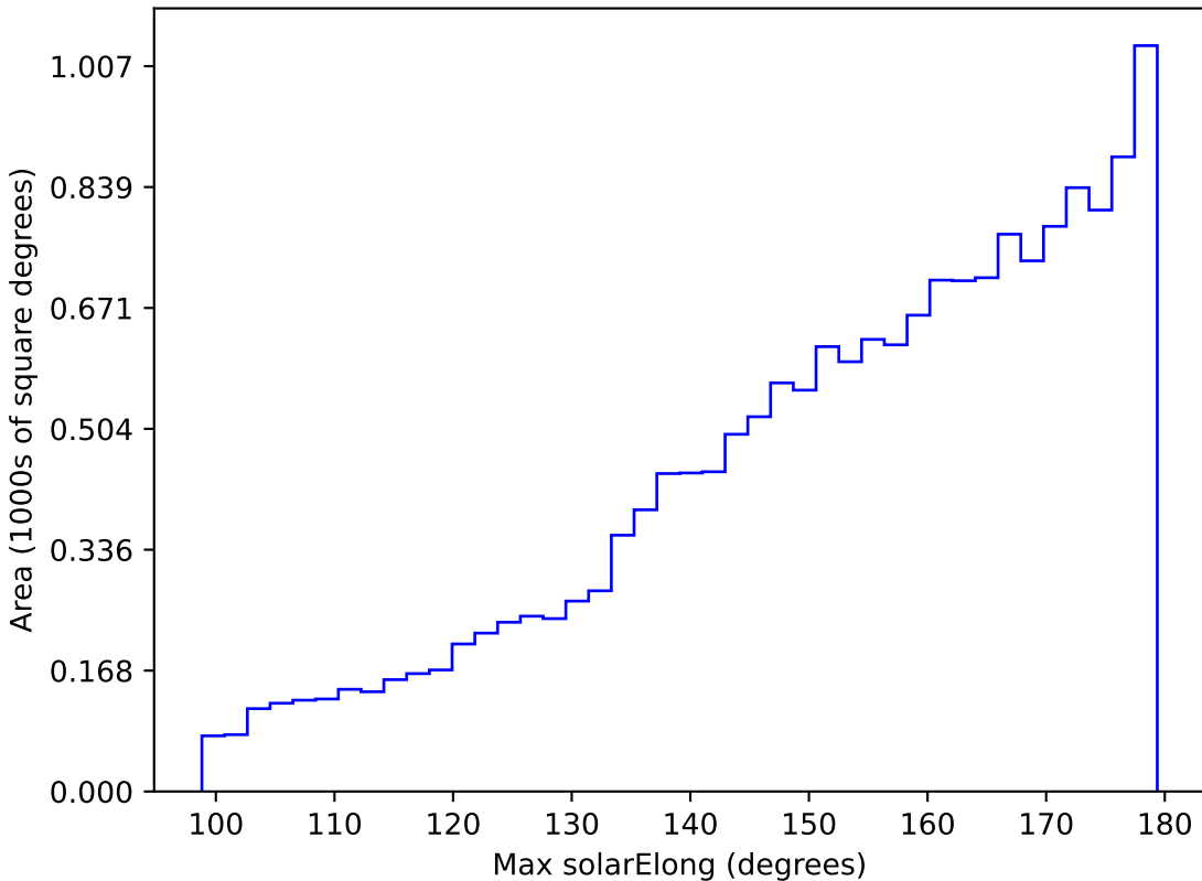
no_magell_roll_v3.4_10yrs WFD z band: Max solarElong
