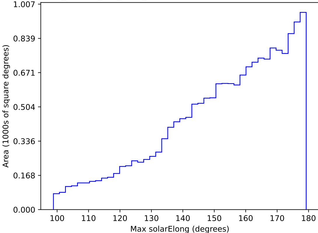
no_magell_roll_v3.4_10yrs WFD y band: Max solarElong
