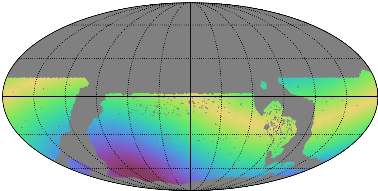
no_magell_roll_v3.4_10yrs WFD u band: Max solarElong
