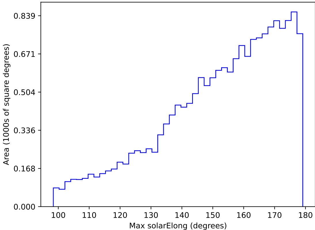
no_magell_roll_v3.4_10yrs WFD u band: Max solarElong
