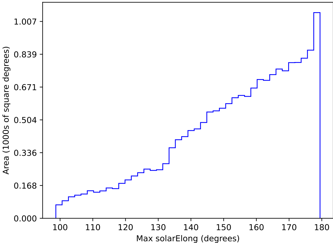
no_magell_roll_v3.4_10yrs WFD r band: Max solarElong
