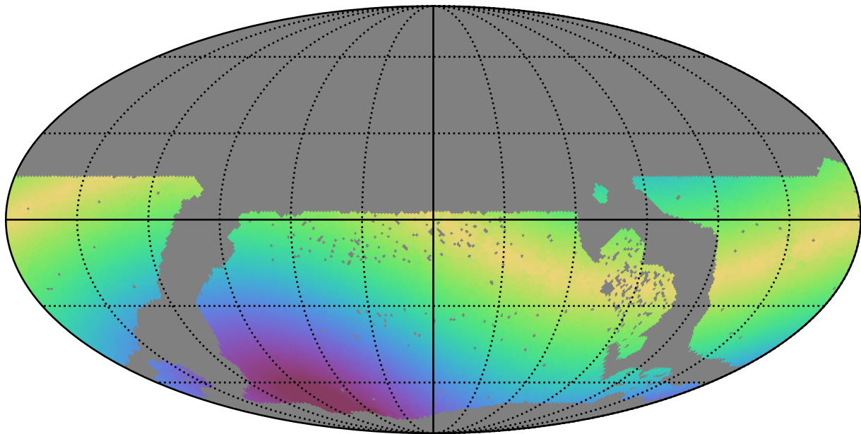
no_magell_roll_v3.4_10yrs WFD g band: Max solarElong
