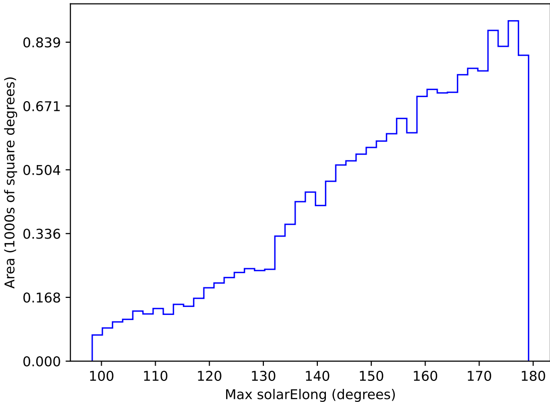
no_magell_roll_v3.4_10yrs WFD g band: Max solarElong
