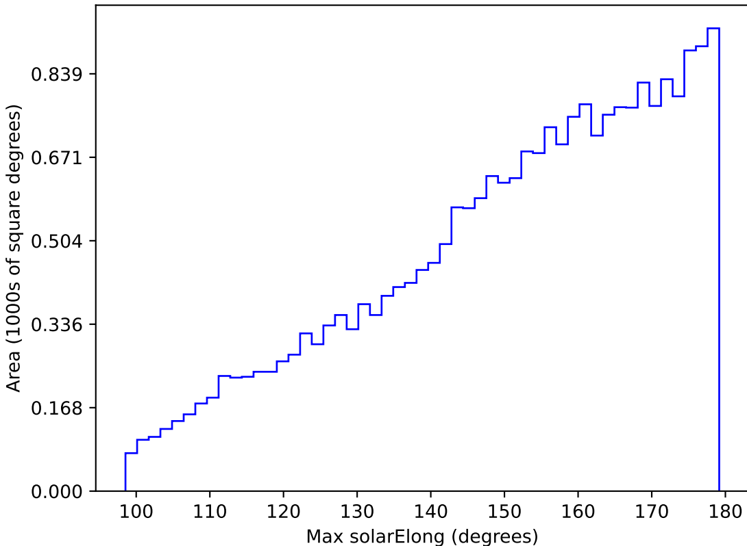
no_magell_roll_v3.4_10yrs All sky y band: Max solarElong
