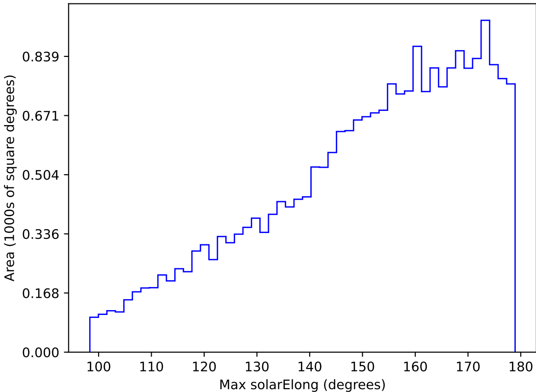
no_magell_roll_v3.4_10yrs All sky u band: Max solarElong
