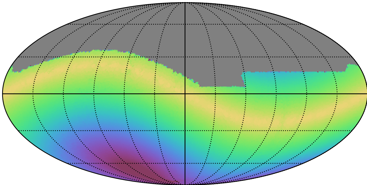
no_magell_roll_v3.4_10yrs All sky r band: Max solarElong
