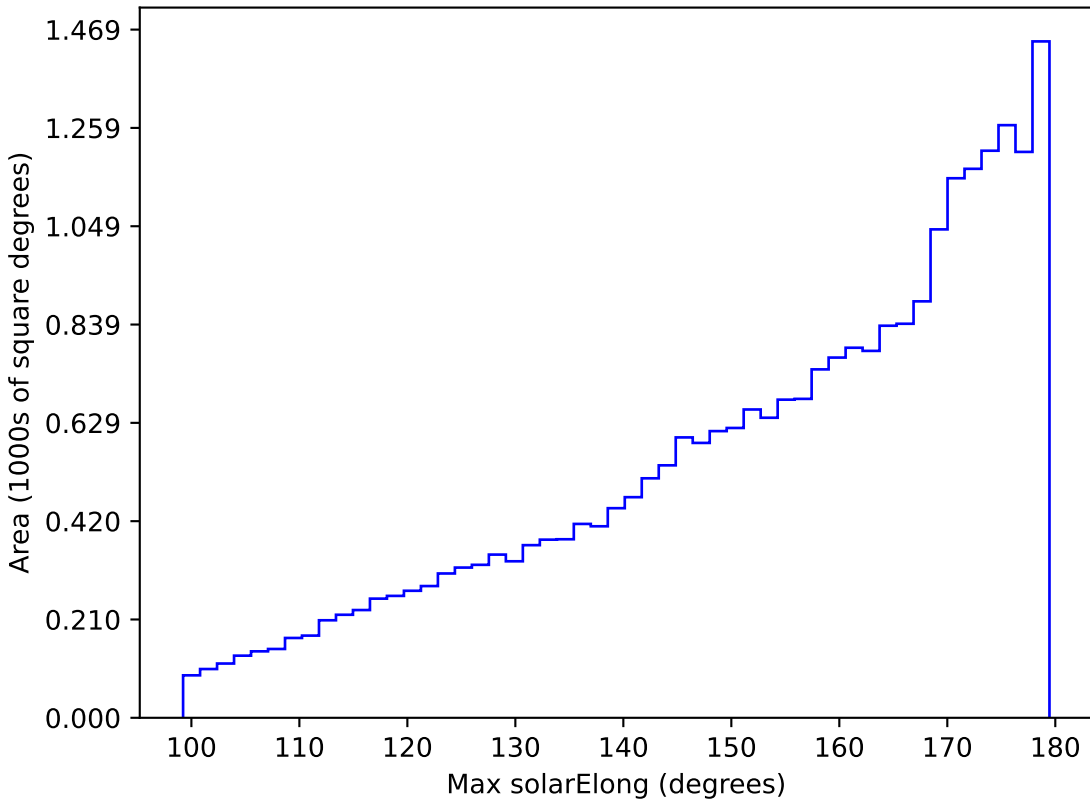
no_magell_roll_v3.4_10yrs All sky r band: Max solarElong
