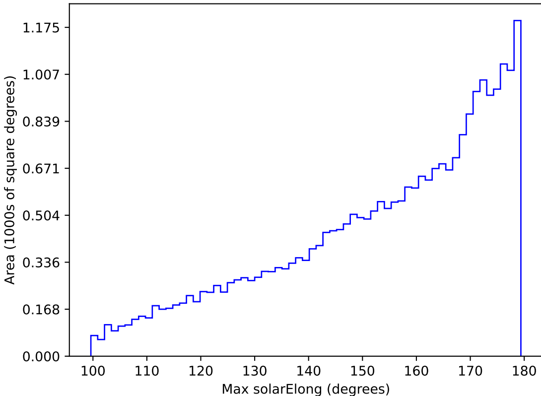
no_magell_roll_v3.4_10yrs All sky i band: Max solarElong
