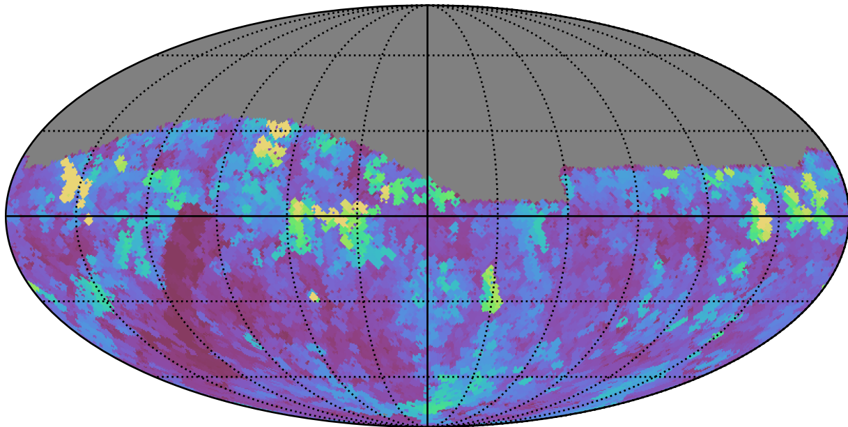
no_magell_roll_v3.4_10yrs Yr 1 z band: Max seeingGeom
