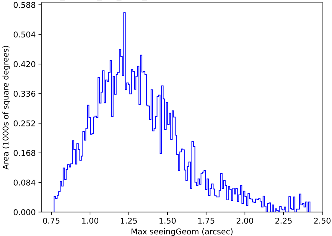
no_magell_roll_v3.4_10yrs Yr 1 i band: Max seeingGeom
