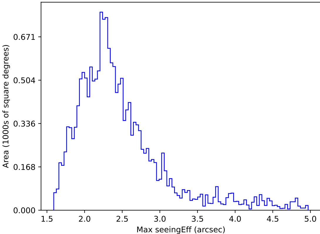
no_magell_roll_v3.4_10yrs WFD y band: Max seeingEff
