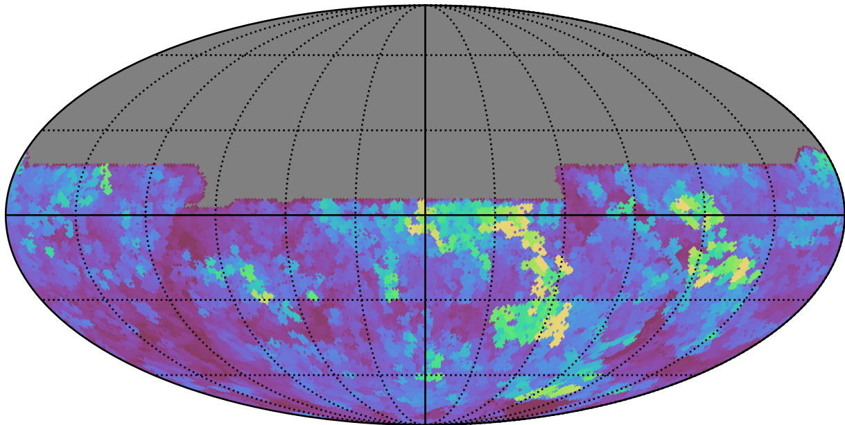
no_magell_roll_v3.4_10yrs All sky y band: Max seeingEff
