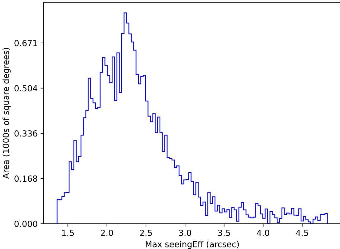
no_magell_roll_v3.4_10yrs All sky y band: Max seeingEff
