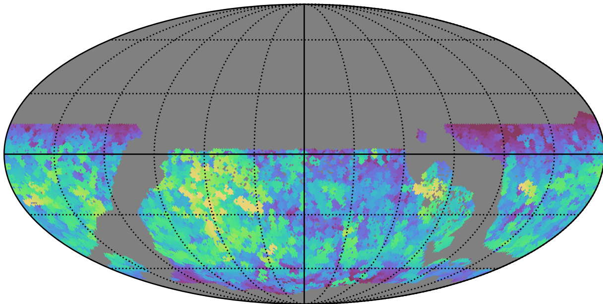
no_magell_roll_v3.4_10yrs WFD z band: Max saturation_mag
