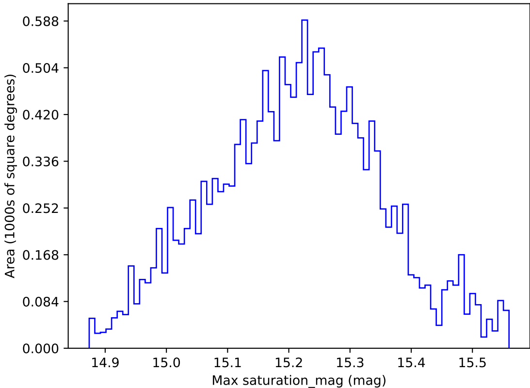
no_magell_roll_v3.4_10yrs WFD z band: Max saturation_mag
