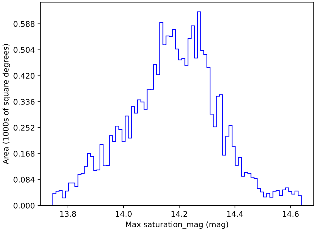
no_magell_roll_v3.4_10yrs WFD y band: Max saturation_mag
