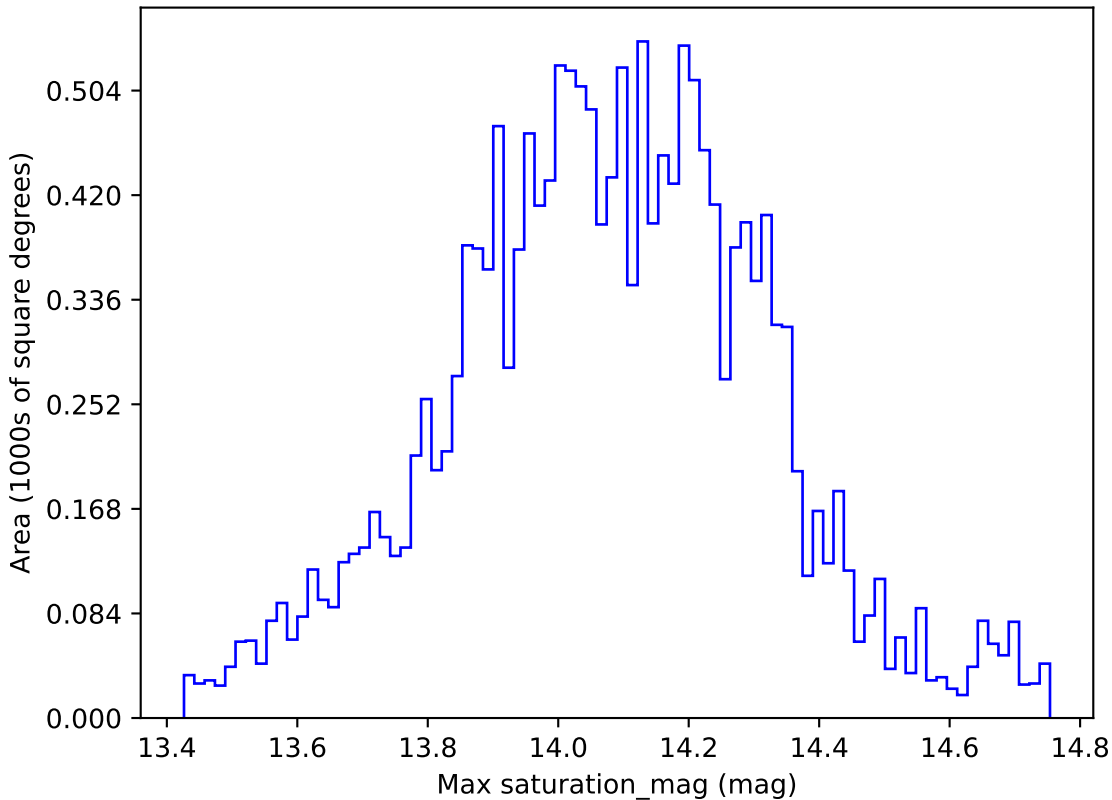
no_magell_roll_v3.4_10yrs WFD u band: Max saturation_mag
