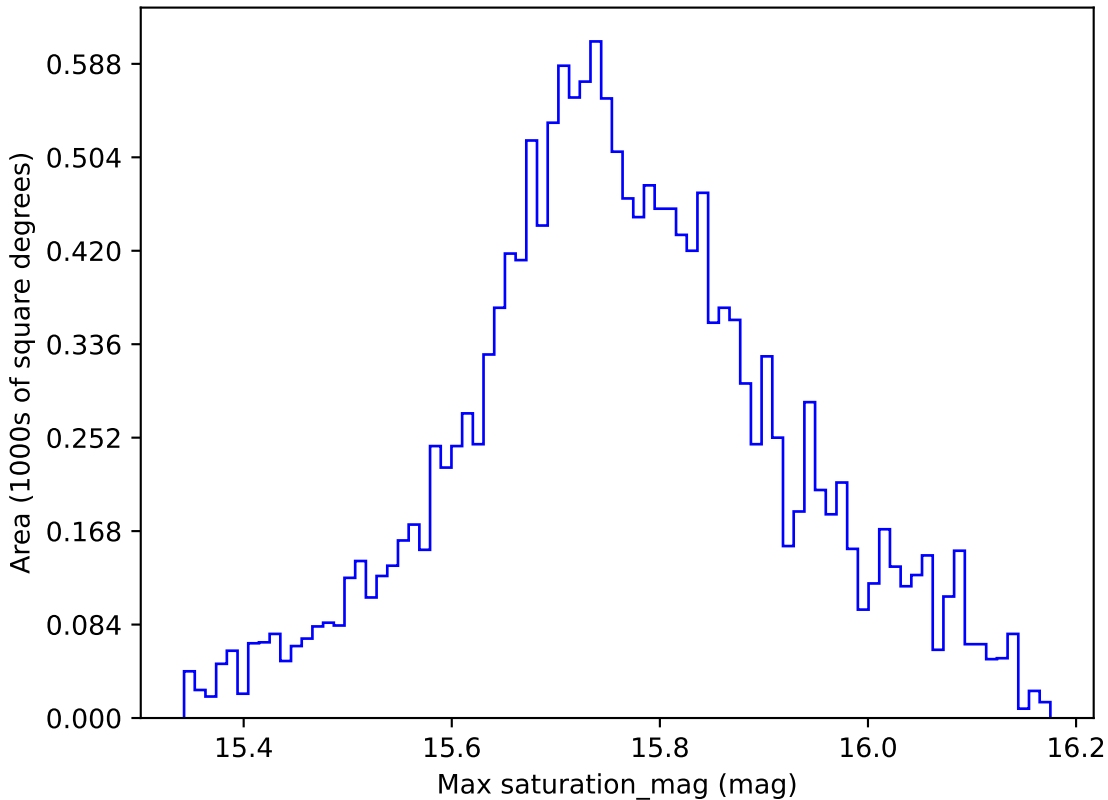
no_magell_roll_v3.4_10yrs WFD r band: Max saturation_mag
