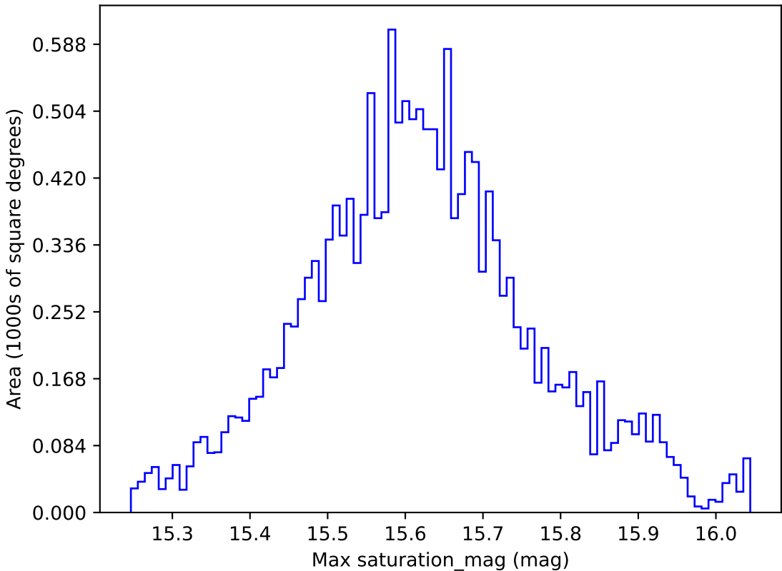
no_magell_roll_v3.4_10yrs WFD i band: Max saturation_mag
