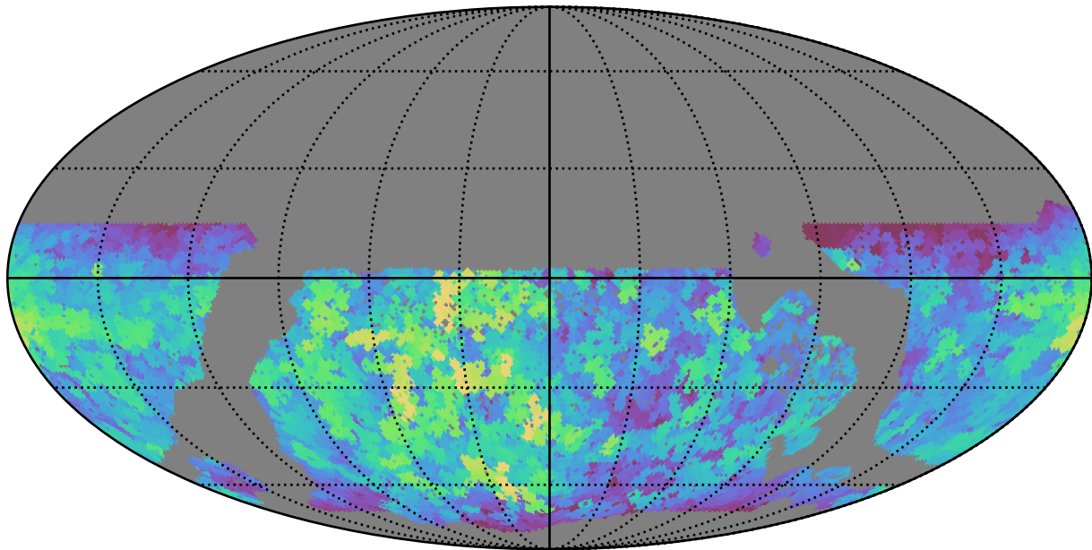
no_magell_roll_v3.4_10yrs WFD g band: Max saturation_mag
