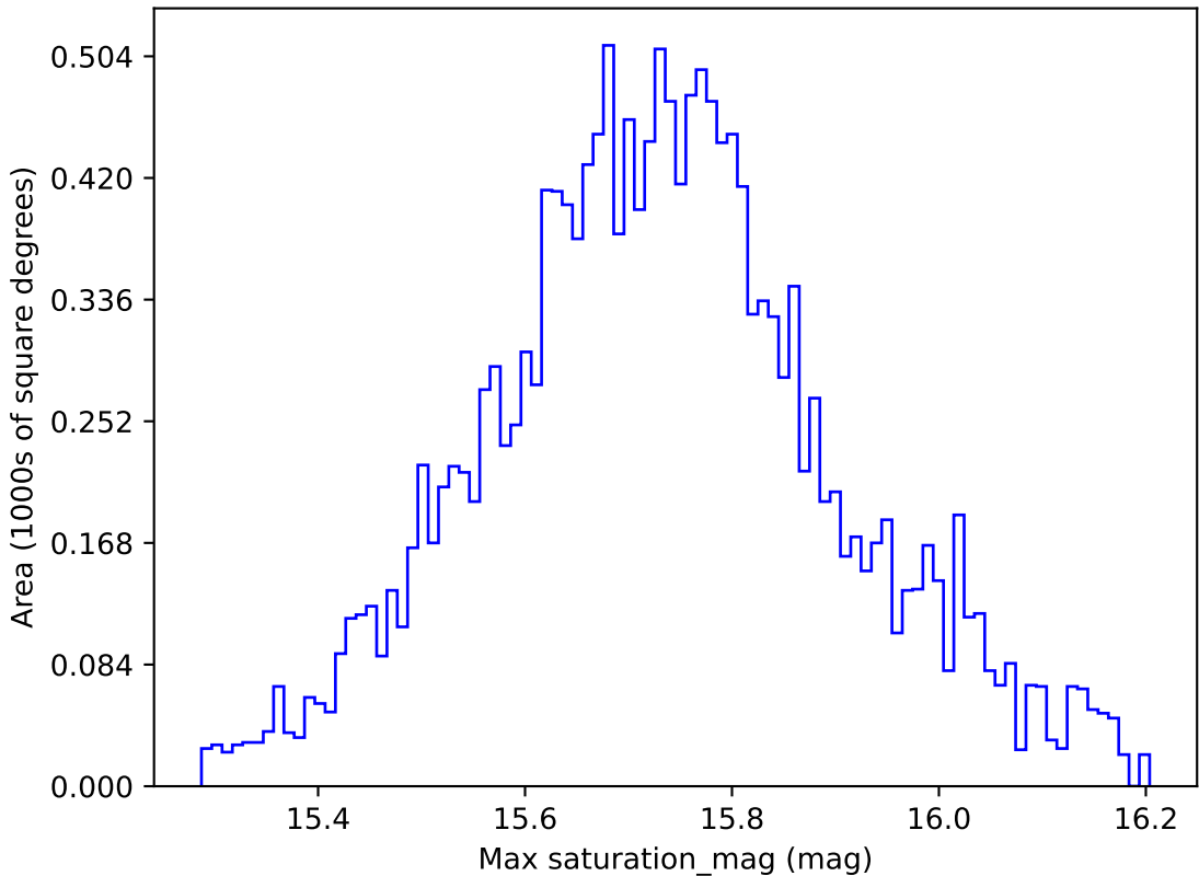
no_magell_roll_v3.4_10yrs WFD g band: Max saturation_mag
