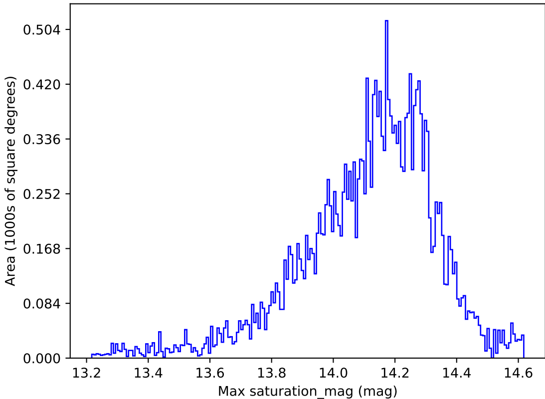
no_magell_roll_v3.4_10yrs All sky y band: Max saturation_mag
